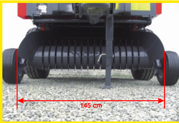
Raccoglitore di larghezza massima 145 cm. Pick-up max width 145 cm.
